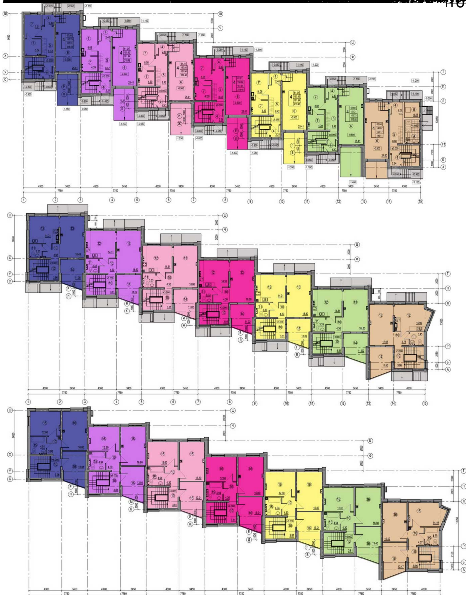
Планировки квартир (таунхаусов) ул. Эстонская, д. 21
